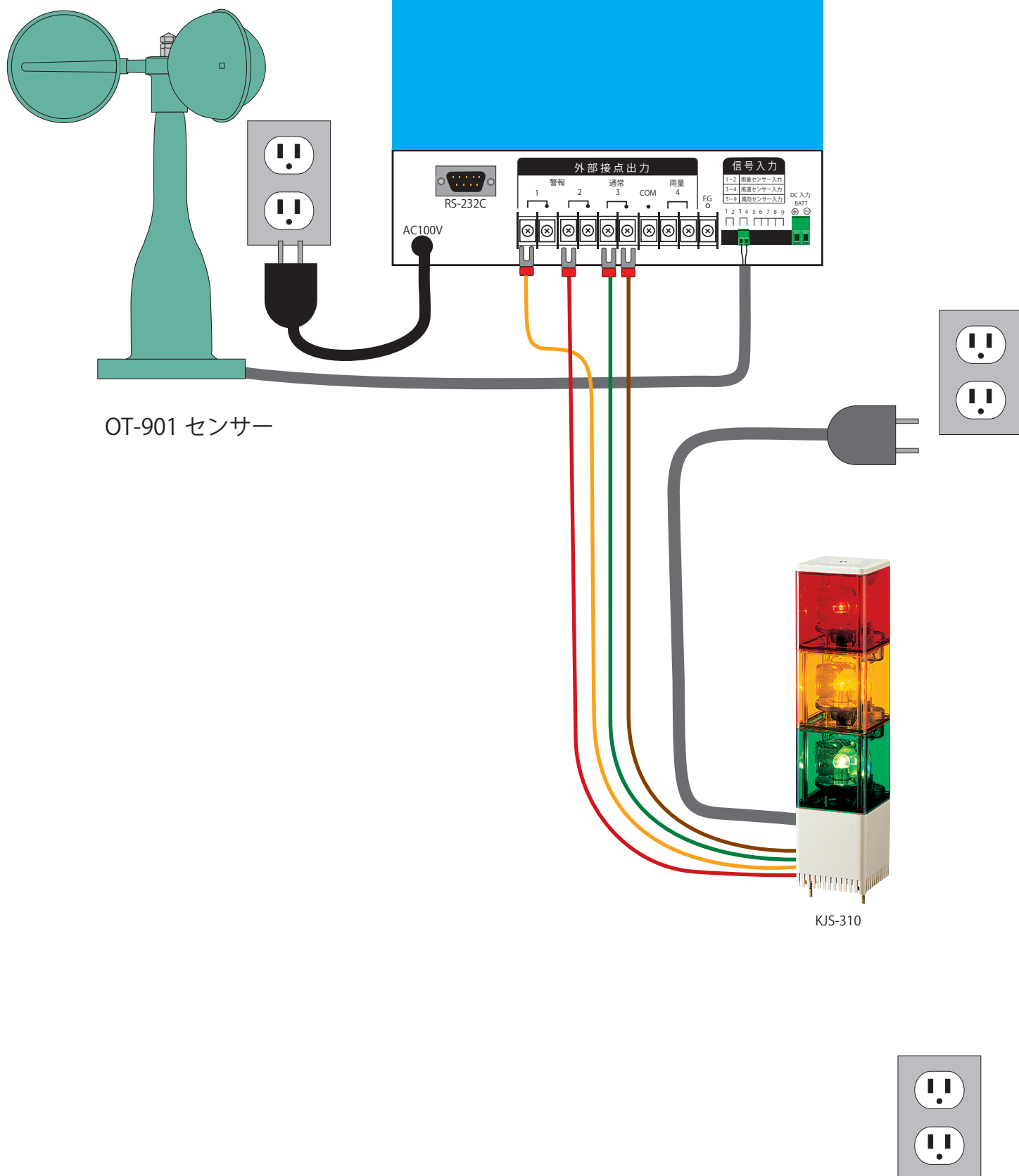
OT-901 ロガー背面
